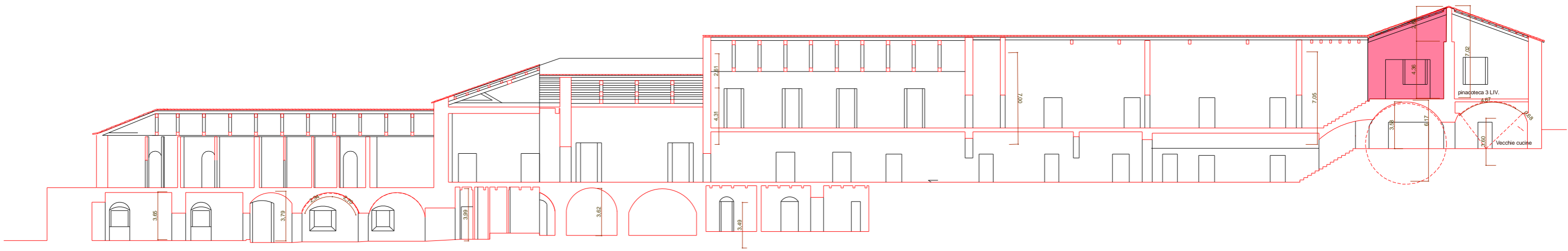
STATO DI FATTO: SEZIONE B-B
