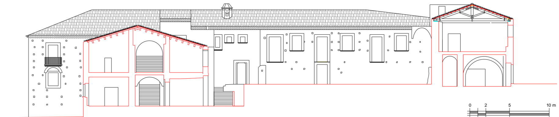
STATO DI FATTO: SEZIONE C-C
