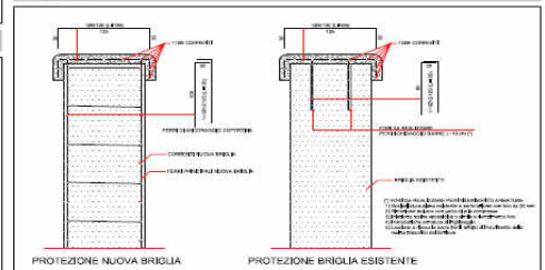
PARTICOLARE COPERTINA IN C.A. - ARMATURE - scala 1:25
