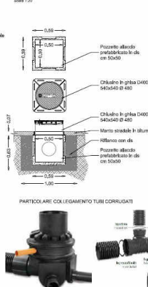
PARTICOLARE POZZETTO DI ALLACCIO IN CALCESTRUZZO Scale 1:20
