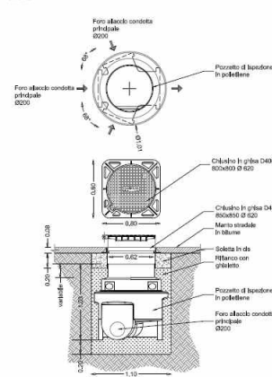
PARTICOLARE POZZETTO DI ISPEZIONE IN POLIETILENE Scale 1:50
