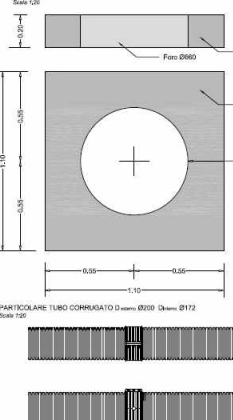
PARTICOLARE SOLETTA IN CALCESTRUZZO COPERTA UNA POZZETTO DI ISPEZIONE Scale 1:20
